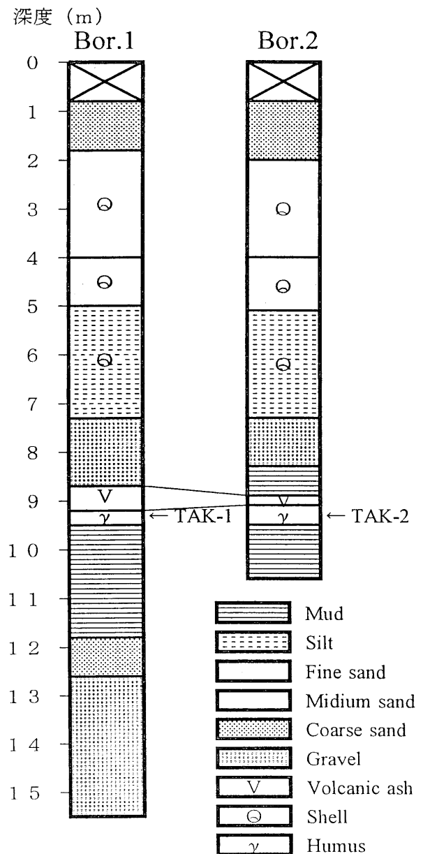
第2図 高松市福岡町ボーリング・コアの層序および年代測定試料採取層準 ←印：年代試料採取層準
